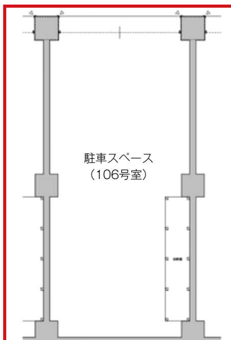
1 階平面図
